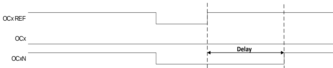
Figure 6.23 延时大于正脉冲宽度的死区波形
