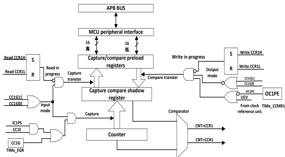
图 6.17 捕获比较通道 1 的主要电路
