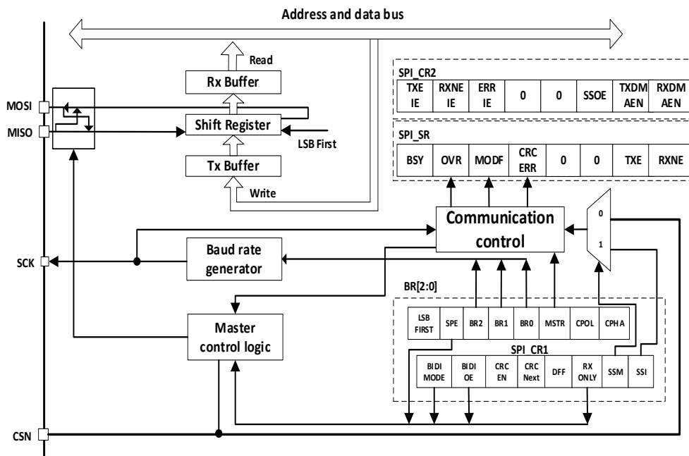
图 6.10 SPI 结构框图
