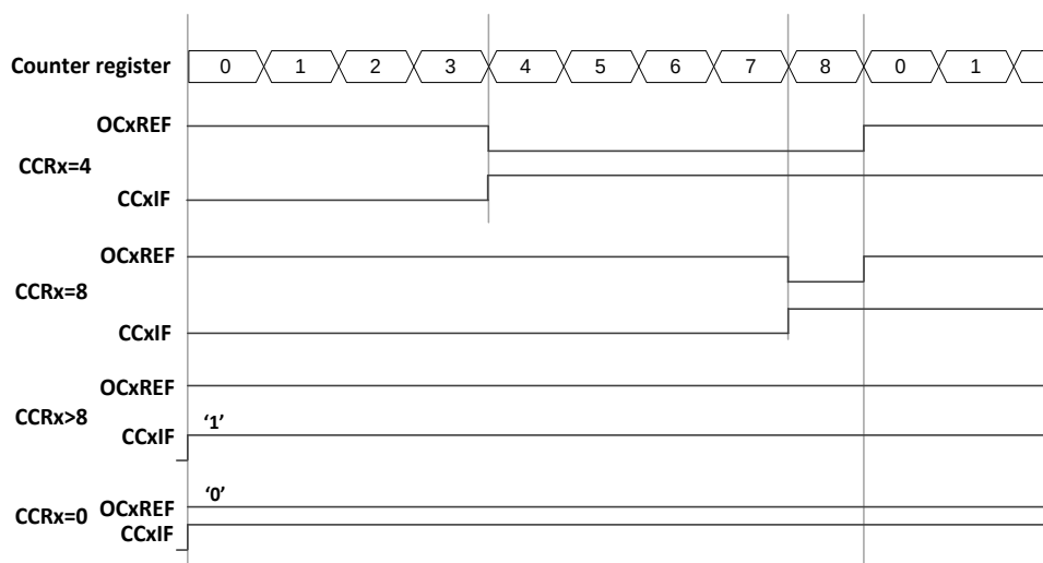
图 6.19 边沿对齐的 PWM 波形 (ARR=8)
