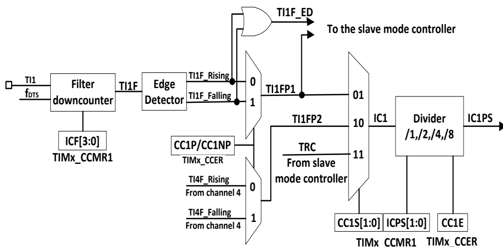
图 6.16 捕获比较通道 (例如: 通道 1 输入阶段)
