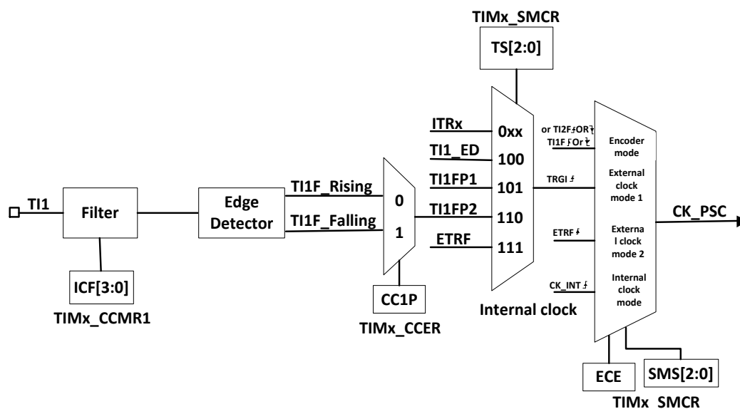
图 6.12 TI1 外部时钟连接实例
