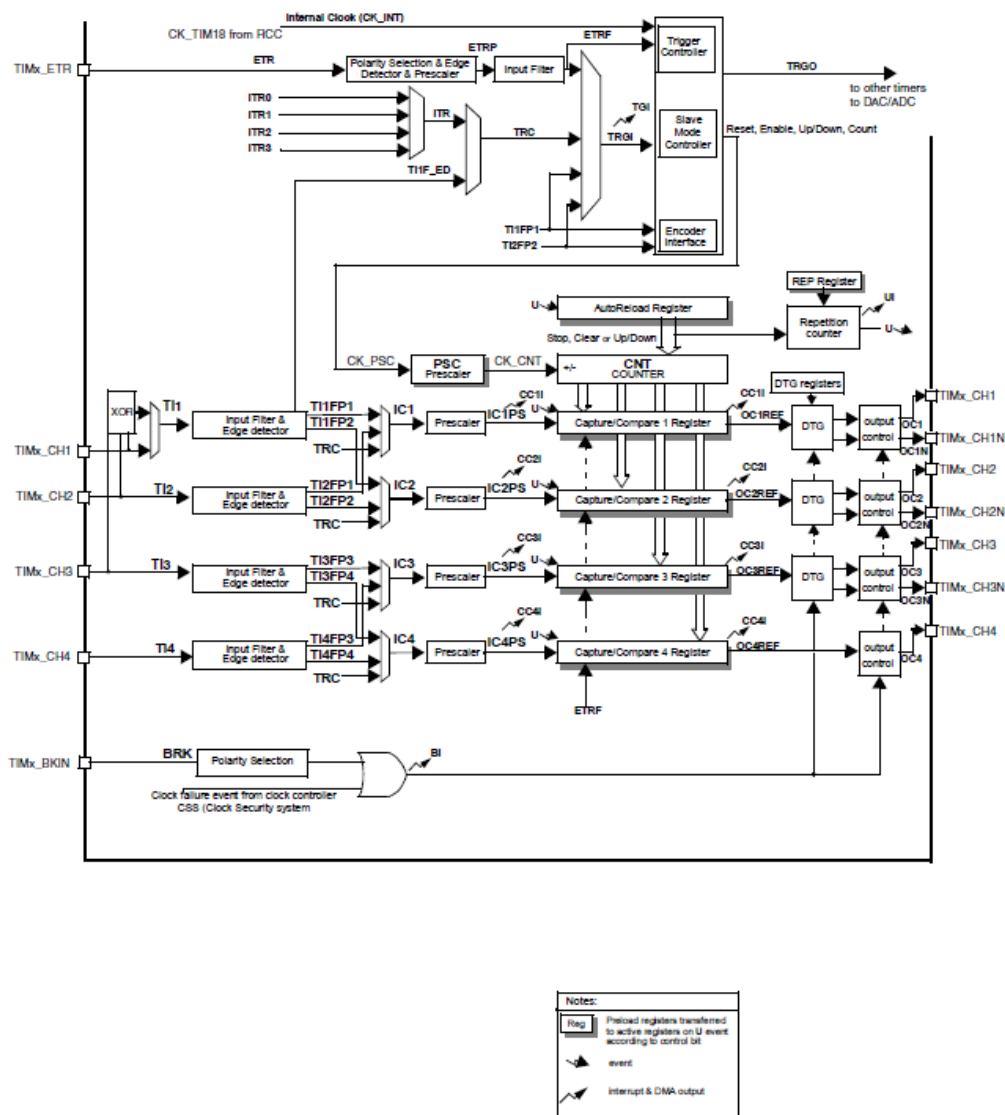
图6.11通用定时器方框图
