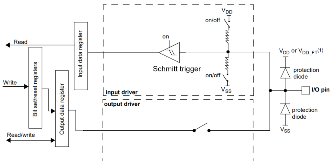
图 6.11 输入的悬空、上拉、下拉配置
