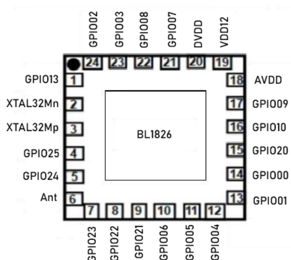
图 2.1BL1826QFN24 管脚定义
