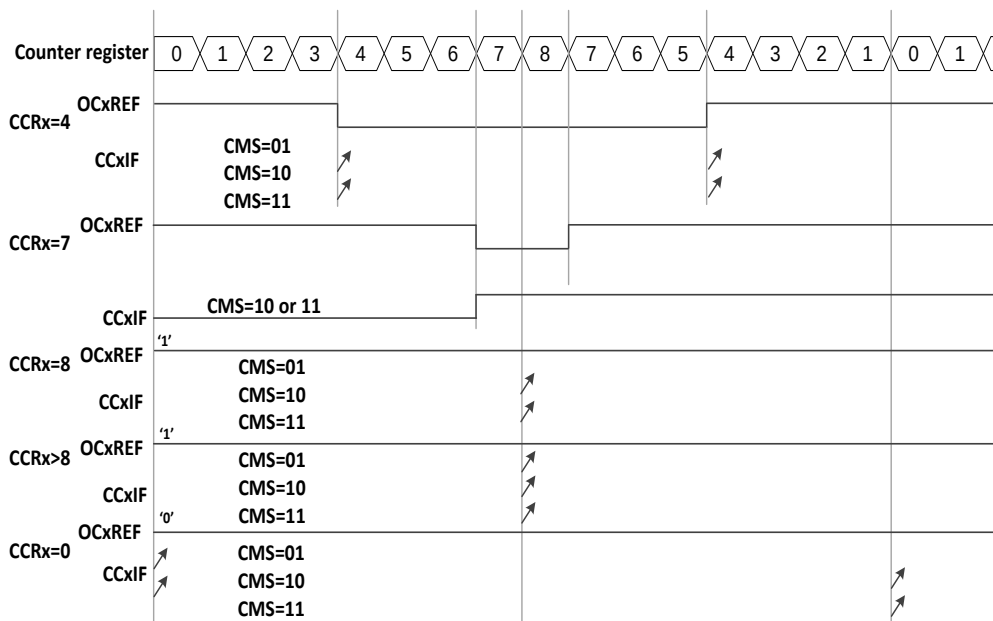
图 6.20 中心对齐的 PWM 波形 (ARR=8)
