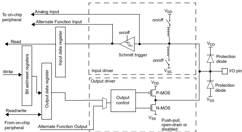
图 6.10 标准 I/O 端口位的基本结构
