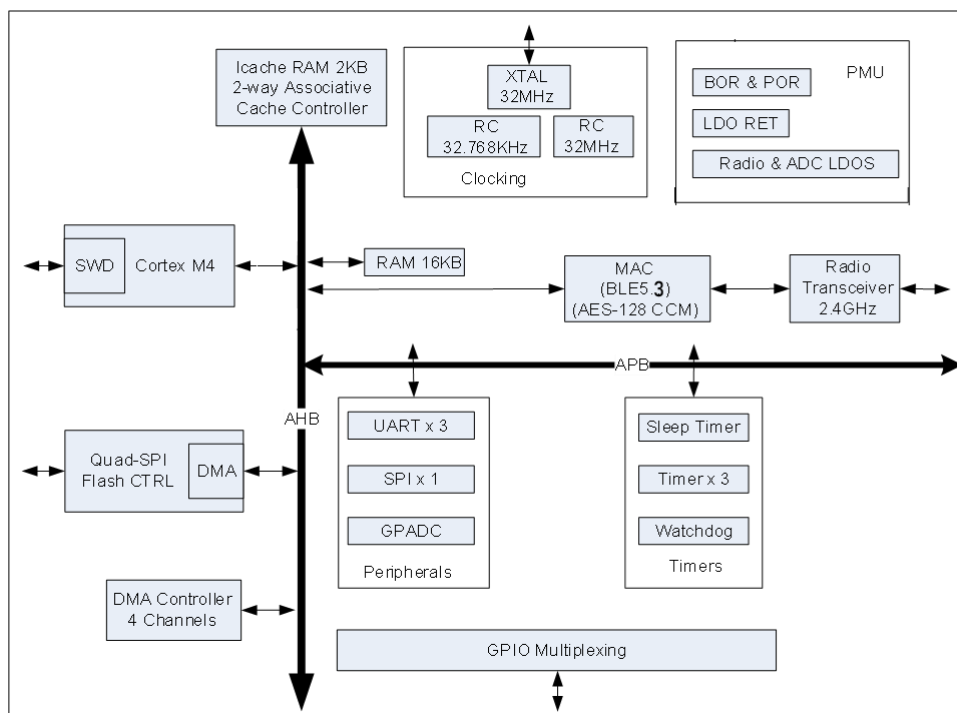
图 1.1BL1826 系统框图
