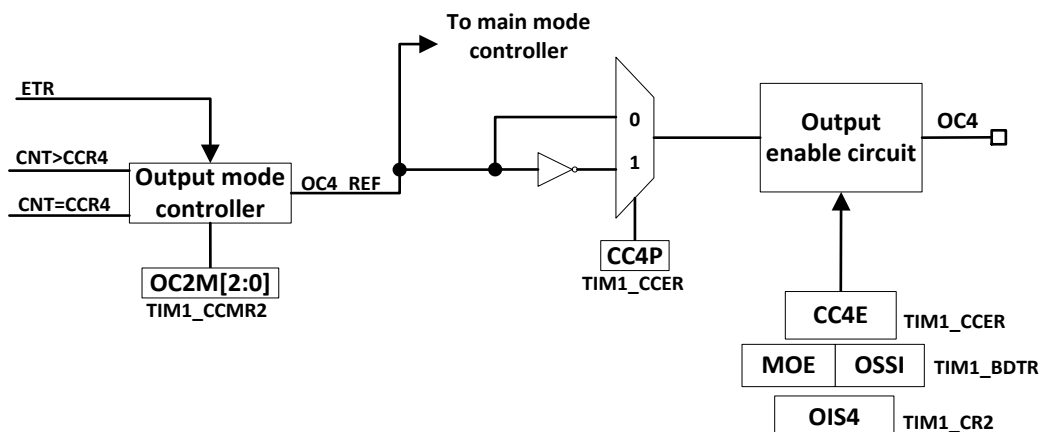
图 6.18 捕获比较器的通道输出部分(通道 4)
