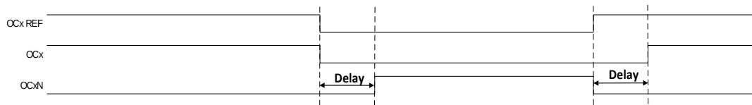
图 6.21 互补输出和死区插入
