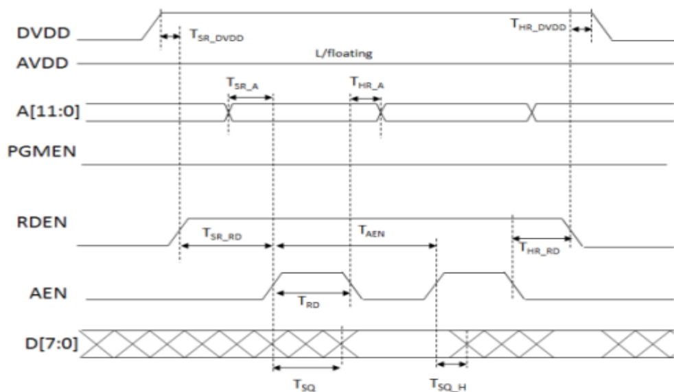
Figure 6.8 读取模式时序图
