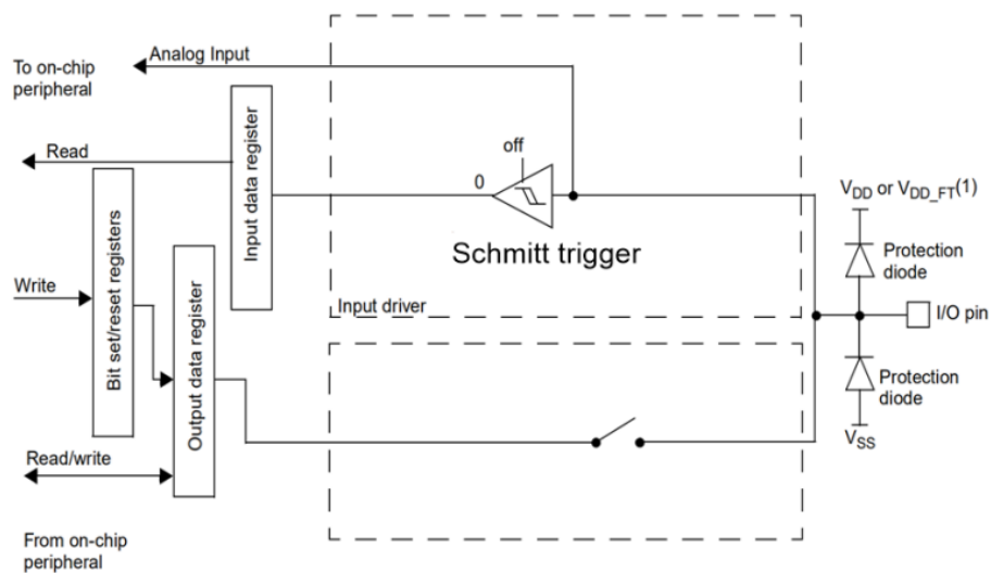
图 6.13 高阻抗-模拟配置
