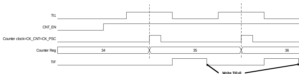
图 6.13 外部时钟模式 1 的控制时序
