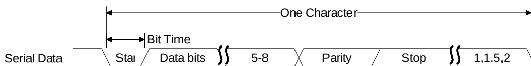
Figure 6.84 串行数据格式
