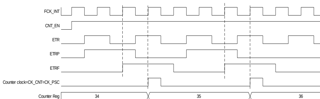
图 6.15 外部时钟模式 2 下的控制时序
