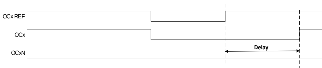
图 6.22 延时大于负脉冲宽度的死区波形
