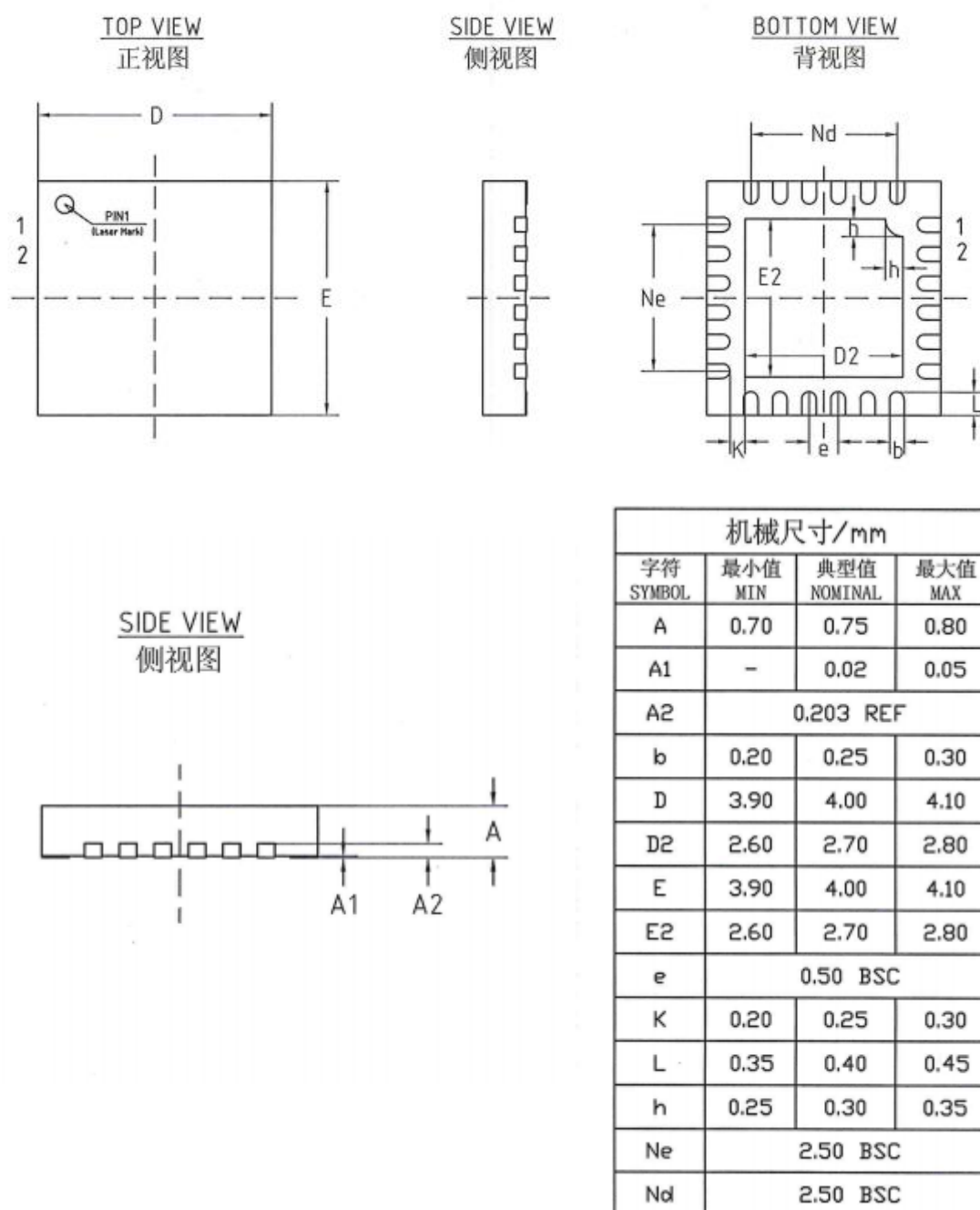
图 9.1BL1826QFN24 封装
